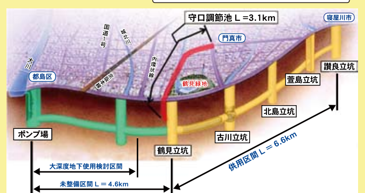
寝屋川北部地下河川 概略図
