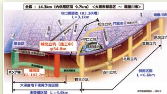
▲ 寝屋川北部地下河川概要図
