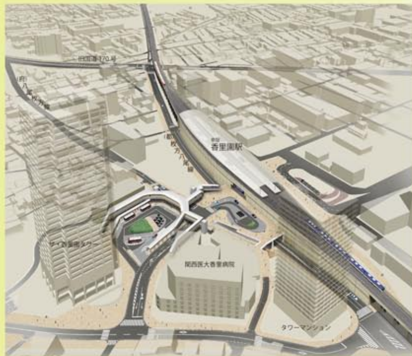
連続立体交差事業完成イメージ図
