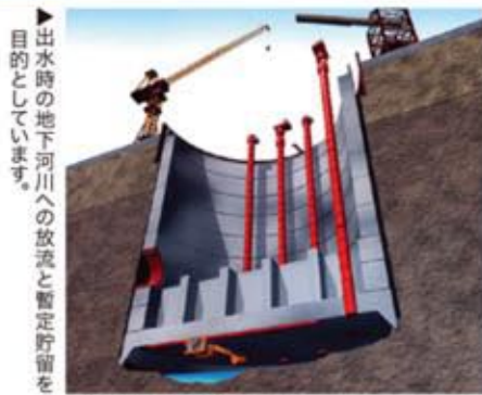
寝屋川市讃良立坑(外径40m、深さ48.8m)
